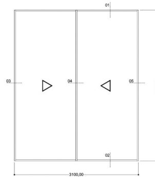
Porta de correr 2 folhas - Sistema Minimalista 3100 x 2400 - Cor: Grafite Perolizado Sl Escala
