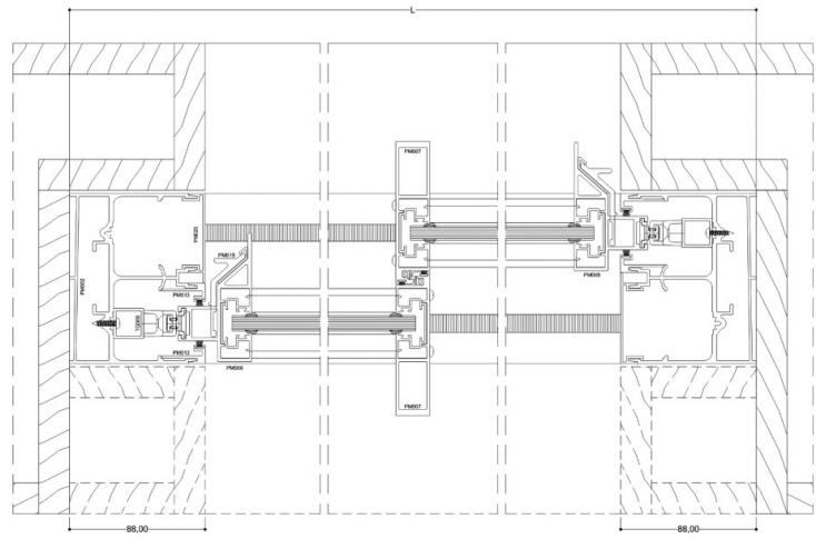
■ Equipamento de madeira a ser instalado: APDS e montagem da encaixote
